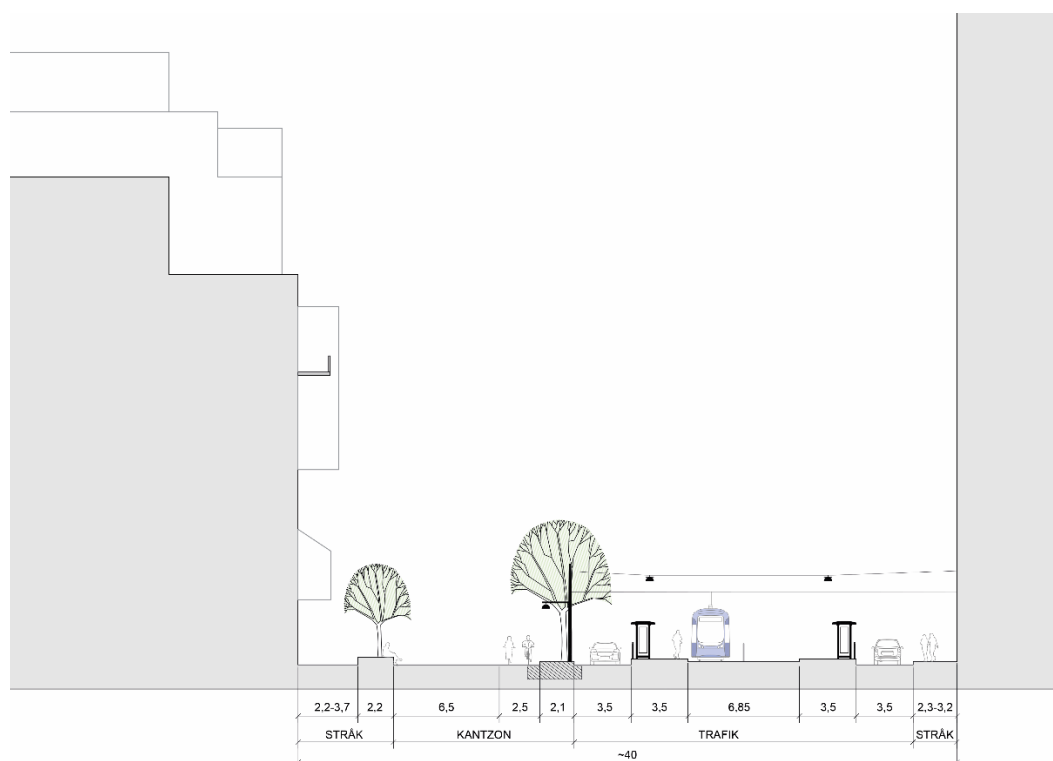
Sektion B-B över en möjlig hållplatsutformning. Skiss AL Studio/02landskap.
